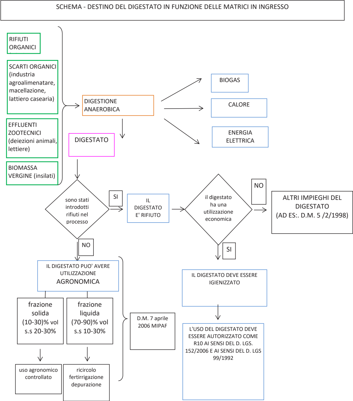
Figura 2 – Schema di flusso che guida l'utilizzo del digestato secondo la normativa.
